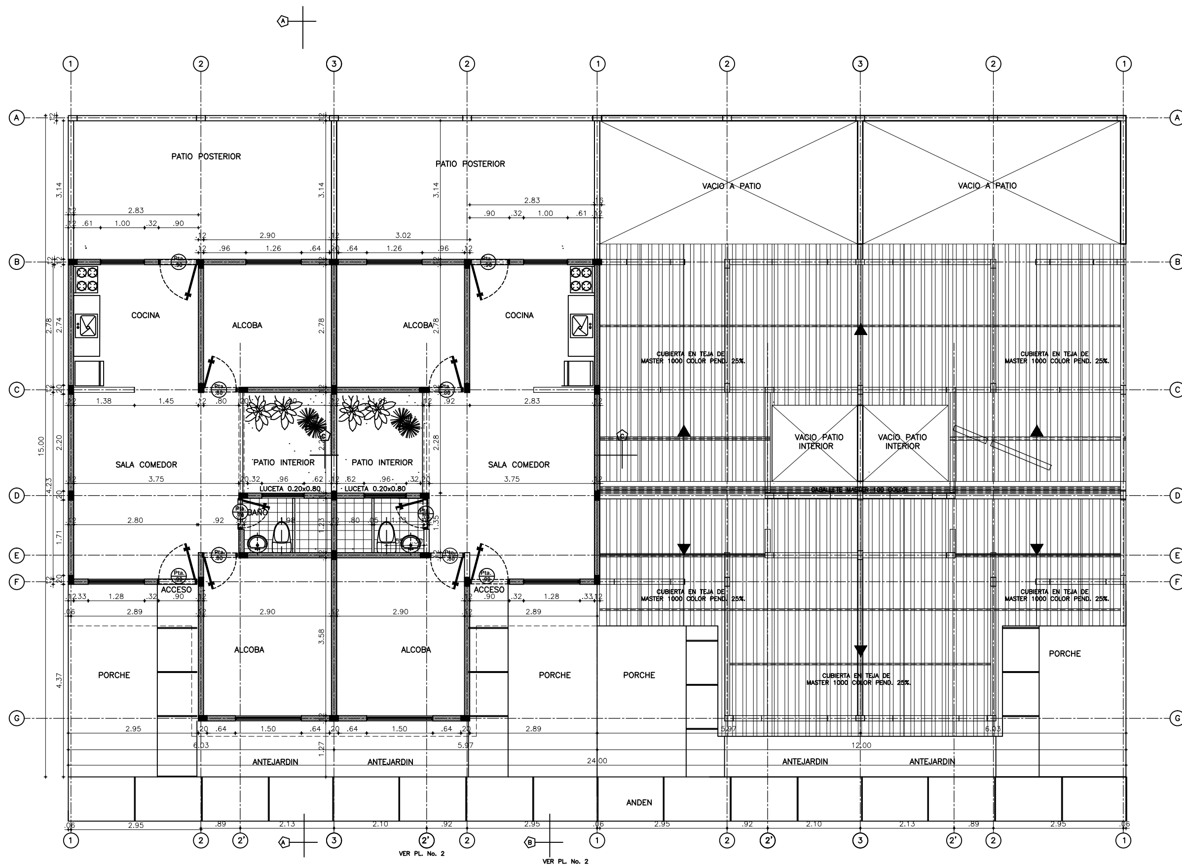
PLANTA ARQUITECTONICA Y DE CUBIERTA MODULO DE CUATRO VIVIENDAS.
